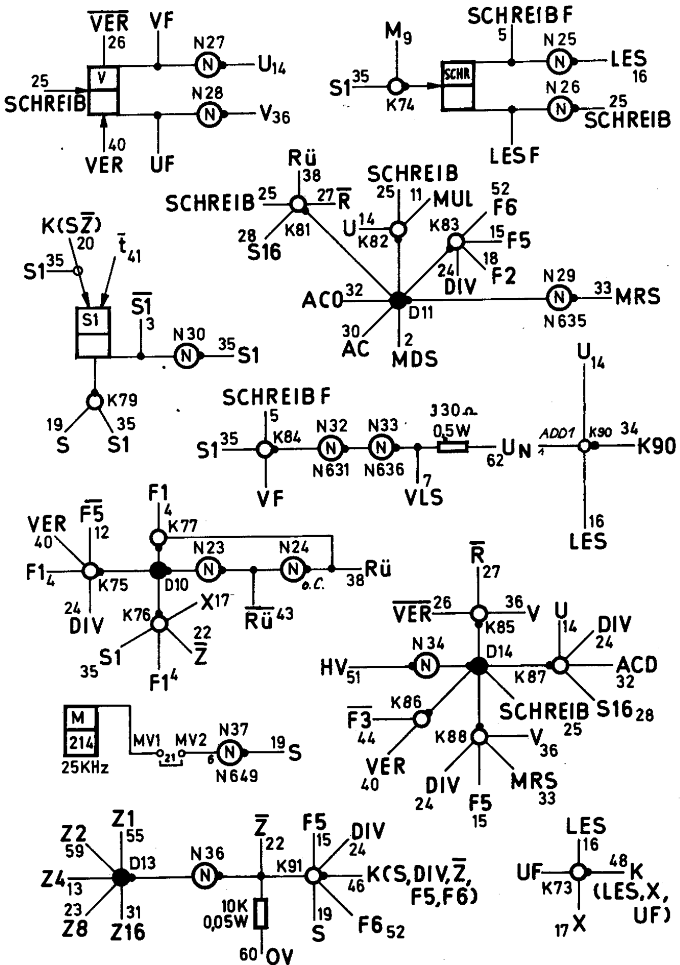
Logischer Plan - Platte 5
