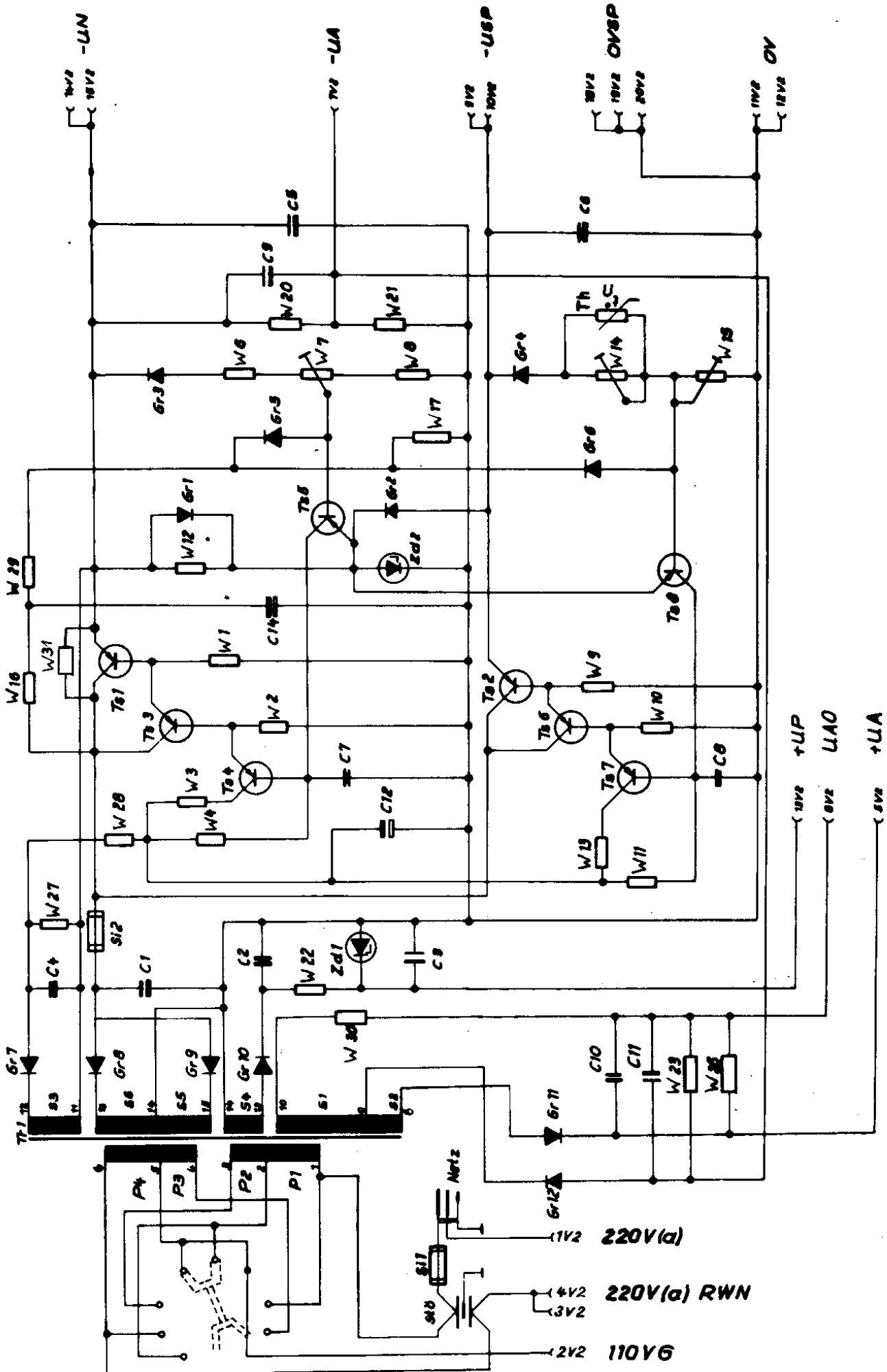
Stromlaufplan - Netzteil 56-220-8000-5
